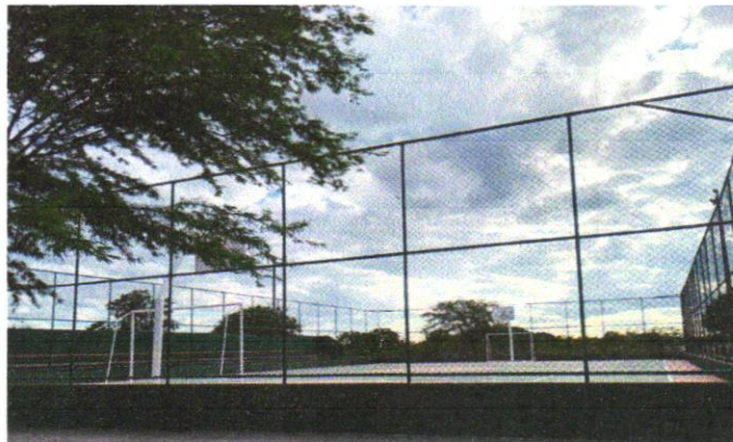
FOTO 01 - ALAMBRADO PARA QUADRA POLIESPORTIVA, ESTRUTURADO POR TUBOS DE AÇO GALVANIZADO, (MONTANTES COM DIAMETRO 2", TRAVESSAS E ESCORAS COM DIÂMETRO 1 1/2"), COM TELA DE ARAME GALVANIZADO, FIO 10 BWG E MALHA
